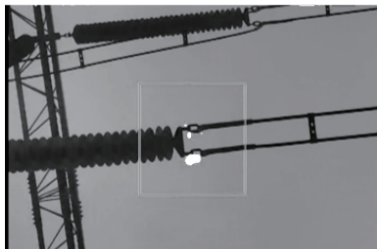
バリ放電
